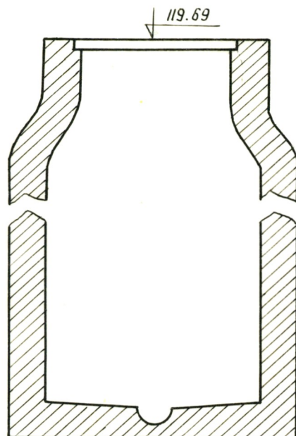
Чертеж колодца М 1:25
