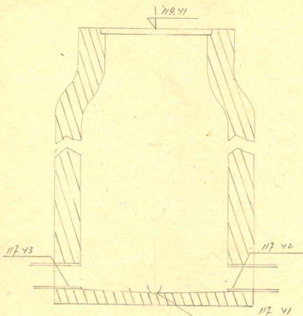
Чертеж колодца М 1:
