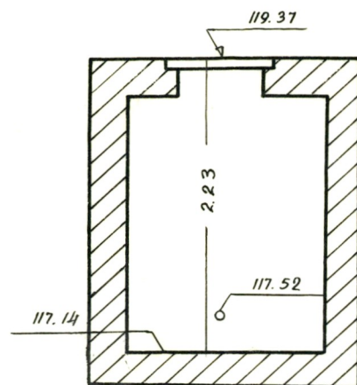
Чертеж колодца М 1:50
