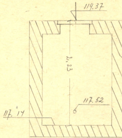
Чертеж колодца М 1:50
