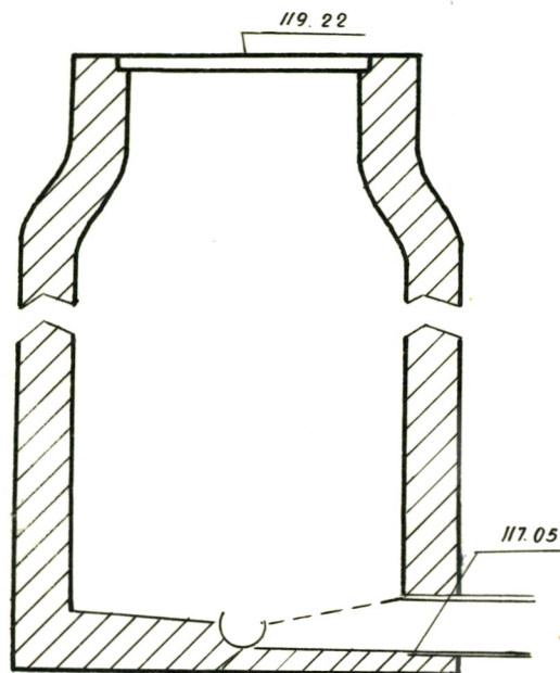
Чертеж колодца М.25
