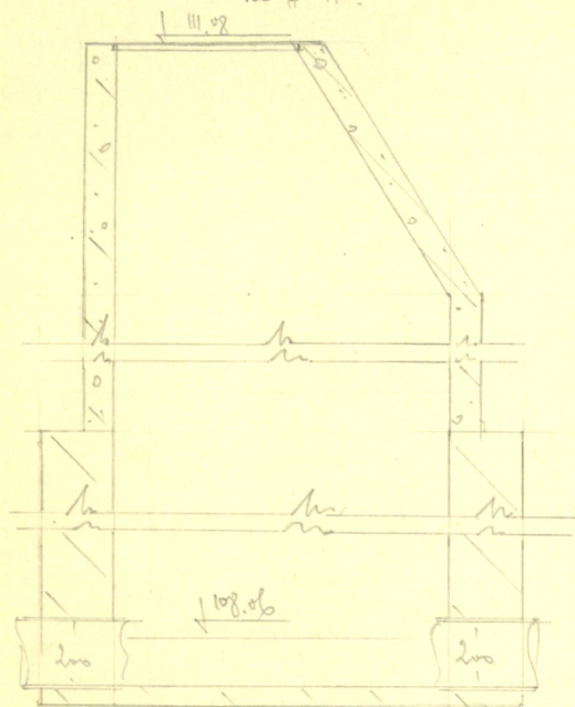
Чертеж колодца М 1:25 по А-А
