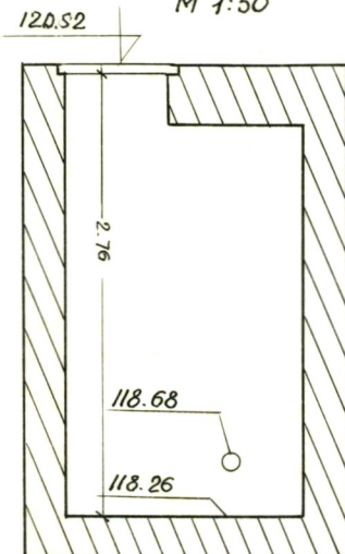
Чертеж колодца М 1:50
