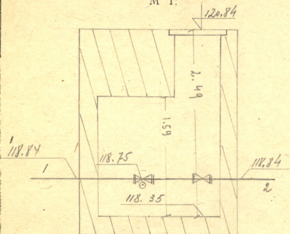
Чертеж колодца М 1.
