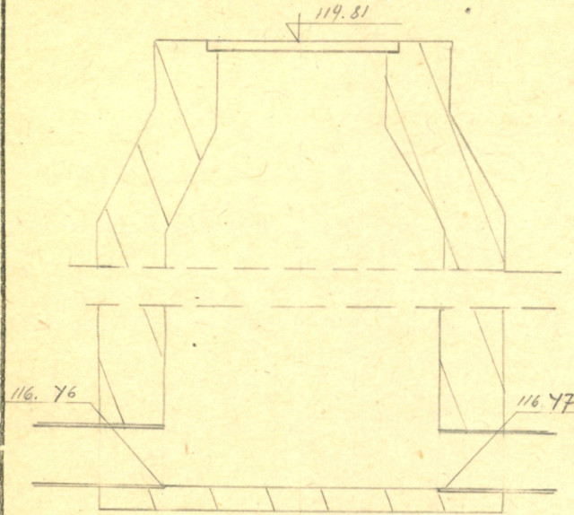
Чертеж колодца М 1:25
