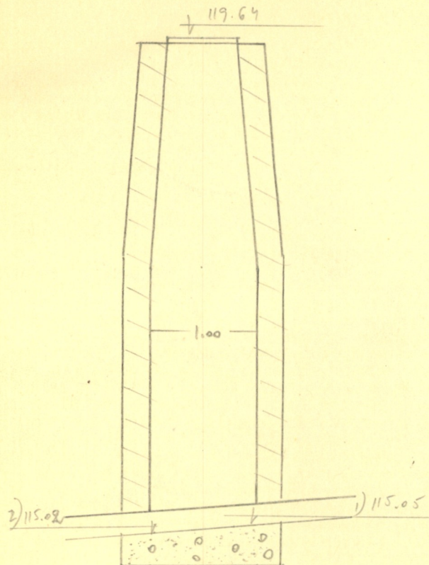
Чертеж колодца М 1:50
