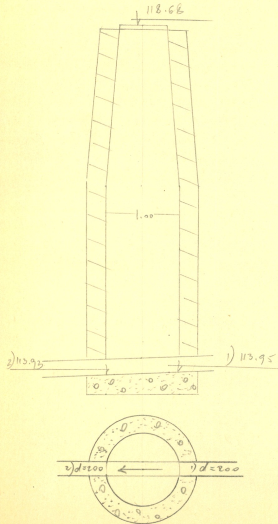
Чертеж колодца М 1:50
