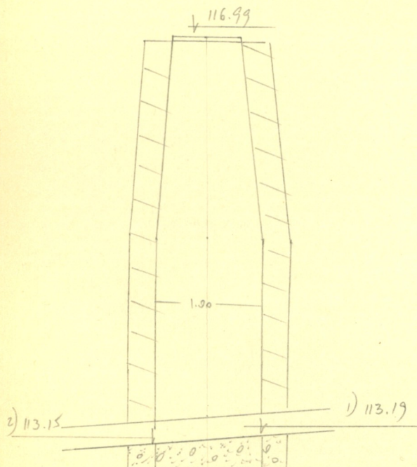
Чертеж колодца М 1:50
