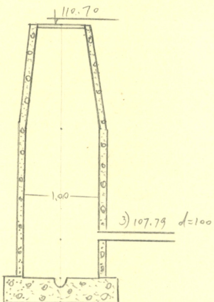
Чертеж колодца М 1:50
