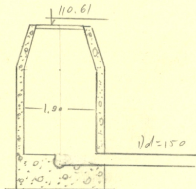
Чертеж колодца М 1:50
