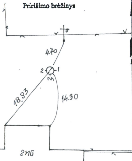
Prirādimo brēžinys
