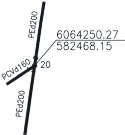
Pririšimo brėžinys
