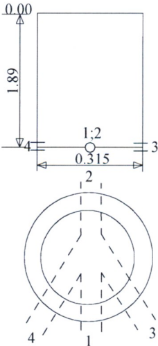
Šulinio pjūviai
