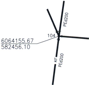
Pririšimo brėžinys
