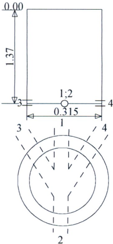
Šulinio pjūviai
