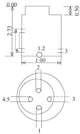
Šulinio pjūviai
