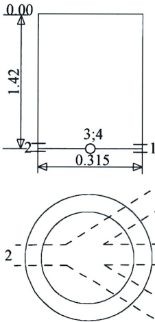
Šulinio pjūviai
