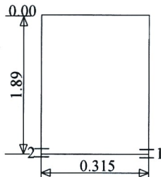
Šulinio pjūviai
