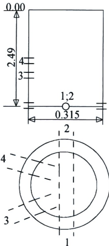
Šulinio pjūviai
