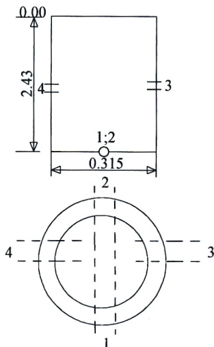
Šulinio pjūviai
