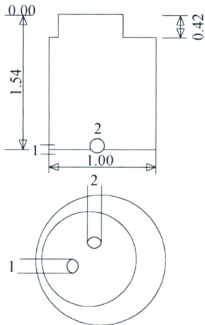
Šulinio pjūviai
