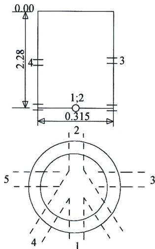
Šulinio pjūviai
