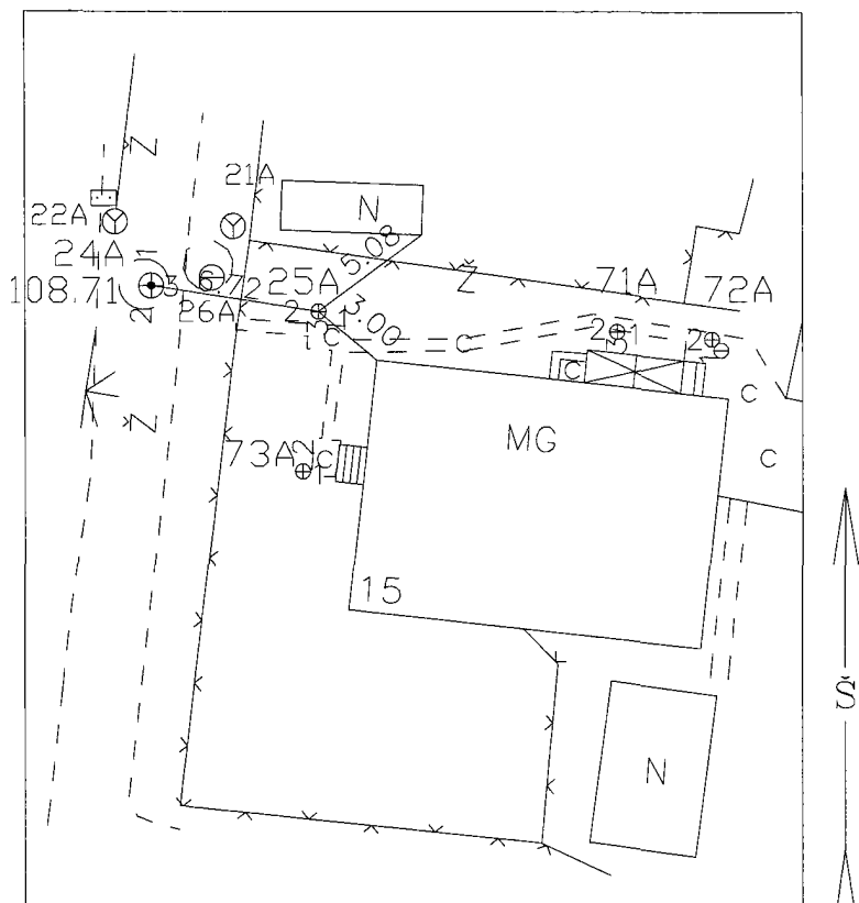
Pririšimo brėžinys :
