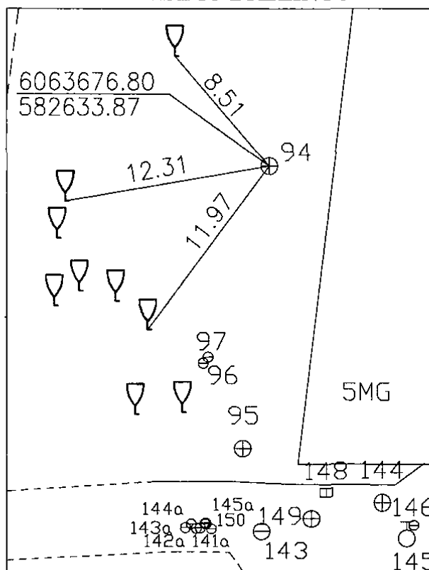
PRIRIŠIMO BRĖŽINYS
