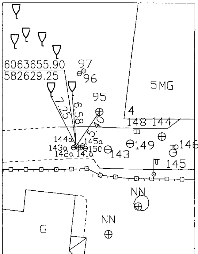
PRIRIŠIMO BRĖŽINYS
