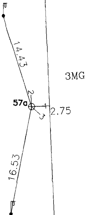
Pririšimo brėžinys
