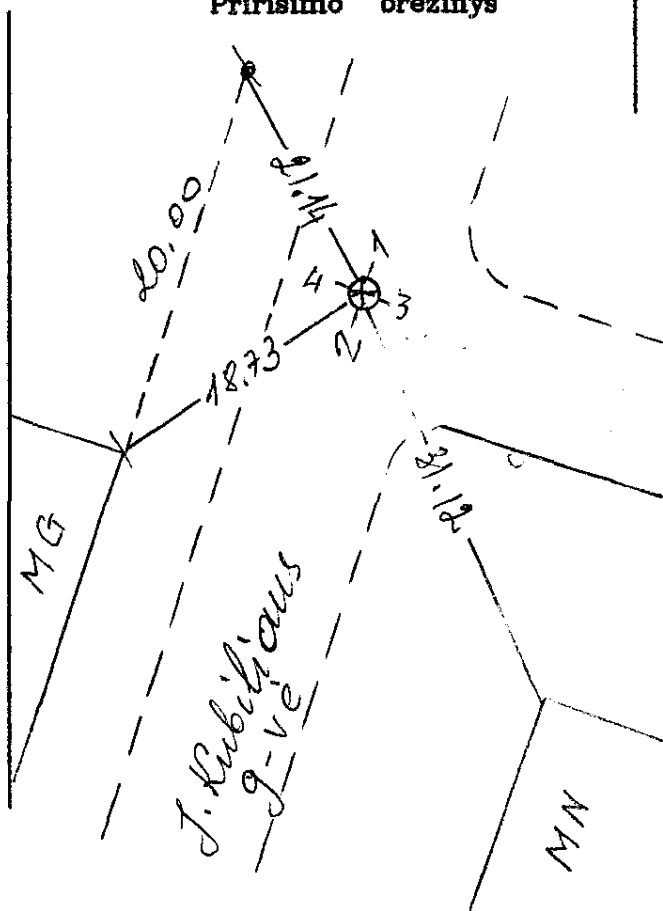
Pririšimo brėžinys
