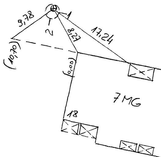
PRIRĖSIMO BRĖŽINYS
