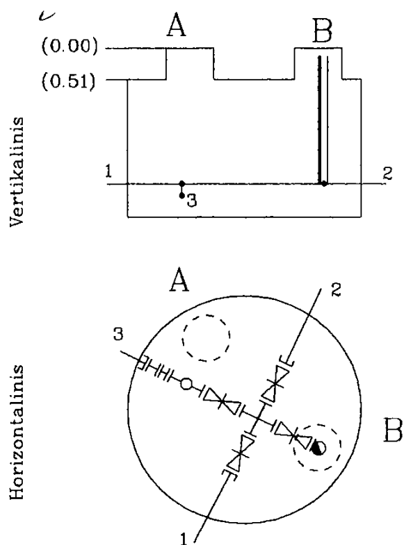
Šulinio pjūviai
