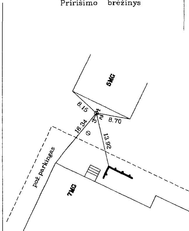
Pririšimo brėžinys
