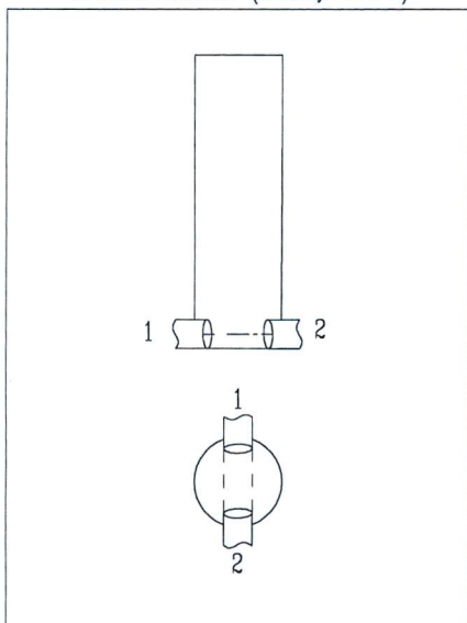
ŠULINIO PŪVIAI (Matmenys duoti m)
