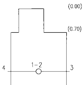
Šulinio pjūviai
