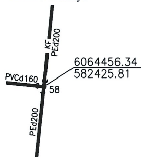
Pririšimo brėžinys
