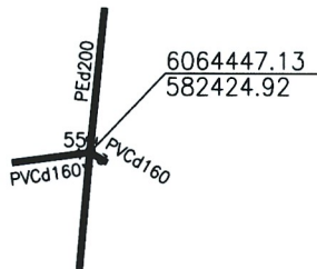
Pririšimo brėžinys
