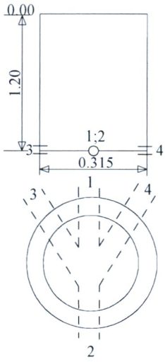
Šulinio pjūviai
