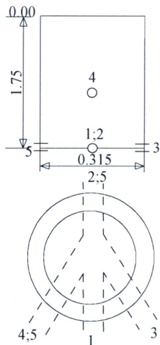
Šulinio pjūviai
