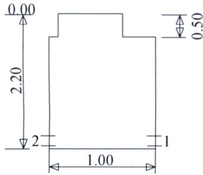
Šulinio pjūviai
