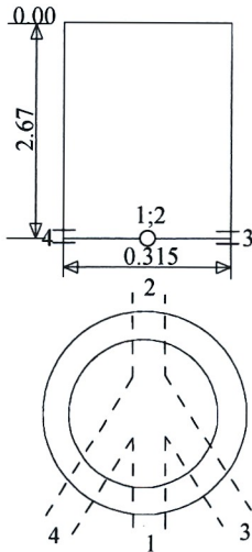
Šulinio pjūviai
