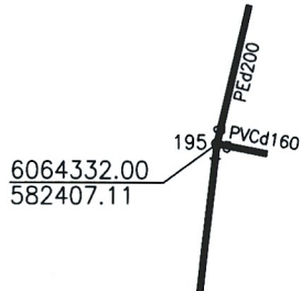
Pririšimo brėžinys
