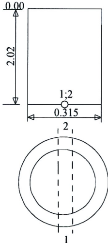
Šulinio pjūviai
