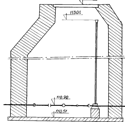
Чертеж колодезя М 1:25
