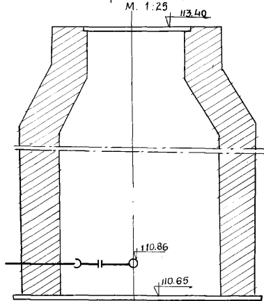
Чертеж колодца
