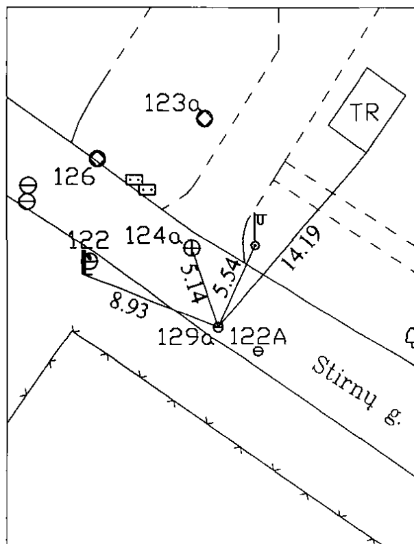
PRIRIŠIMO BRĖŽINYS
