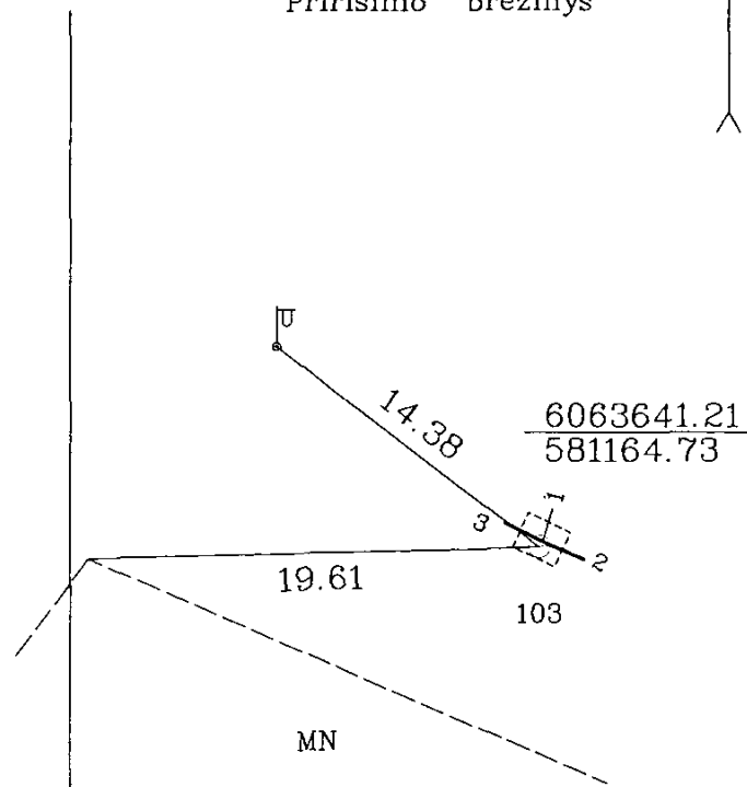
Pririšimo brėžinys
