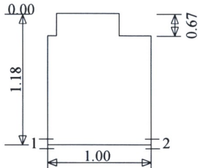
Šulinio pjūviai
