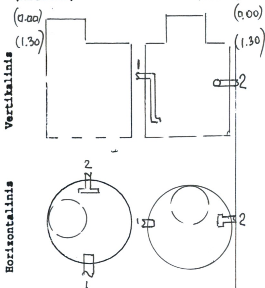
PRIRIŠIMO SCHEMA
