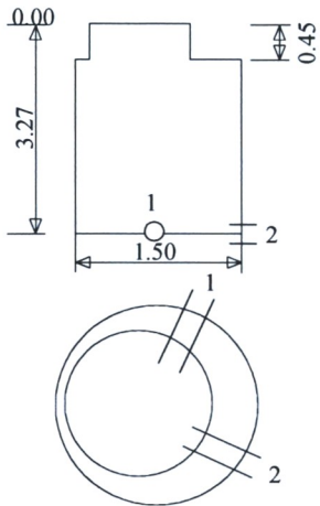
Šulinio pjūviai
